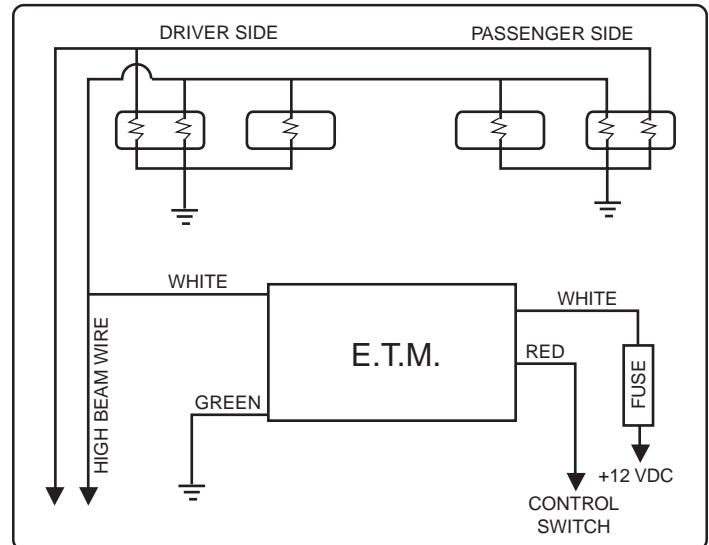
Wiring Schematic
