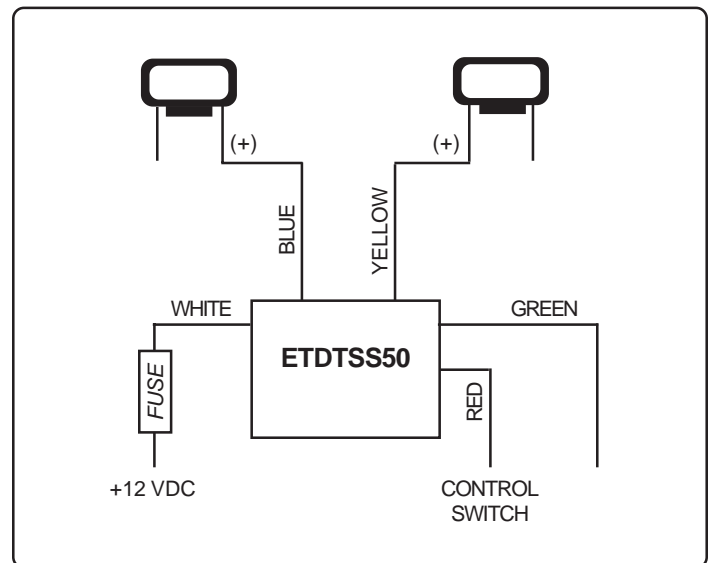
Wiring Schematic
